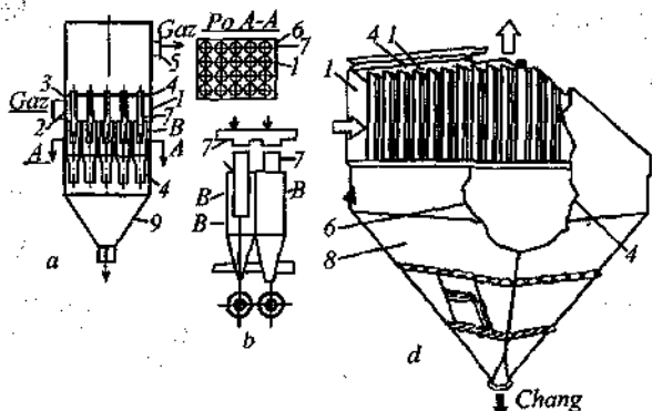
62- rasm. Batareyali siklon:
