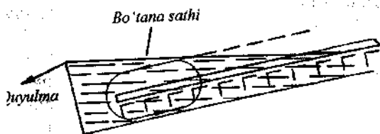
47- rasm. Reykali klassifikatorlarda eshkaklarning harakatlanish sxemasi.
