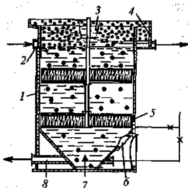
39-rasm. Pnevmatik flotatsiya mashinasi ФП-100: 1—yuklovchi tuynik; 2—ko'pik qaytargich; 3—halqali tarnovcha; 4, 6—aeratorlar; 5—mok; 8—bo'shatish tuynugi.
