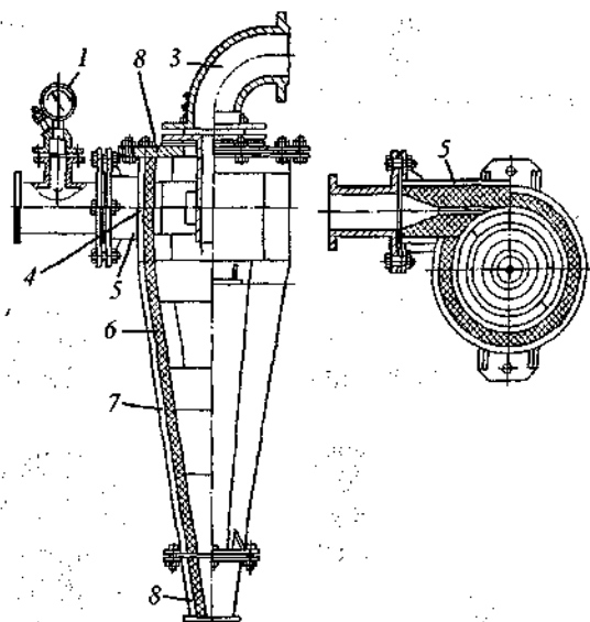
25-rasm. Gidrosiklon:
