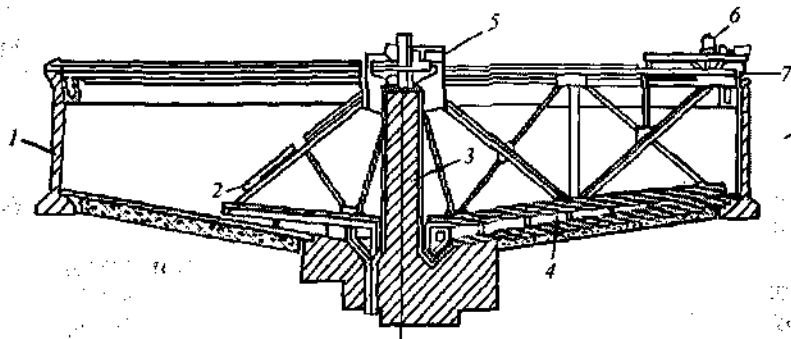
52- rasm. Tashqi uzatmali silindrik quyultirgich: 1—temir betonli hovuz; 2—ferma; 3—markaziy kolonna; 4—eshkakli rama; 5—podshipnik; 6—aravacha; 7—rels.
