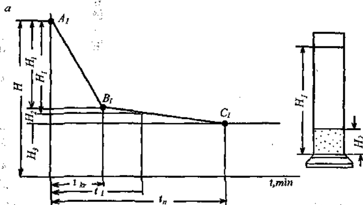
49- rasm. Quyultirish egri chizigʻi grafi.
